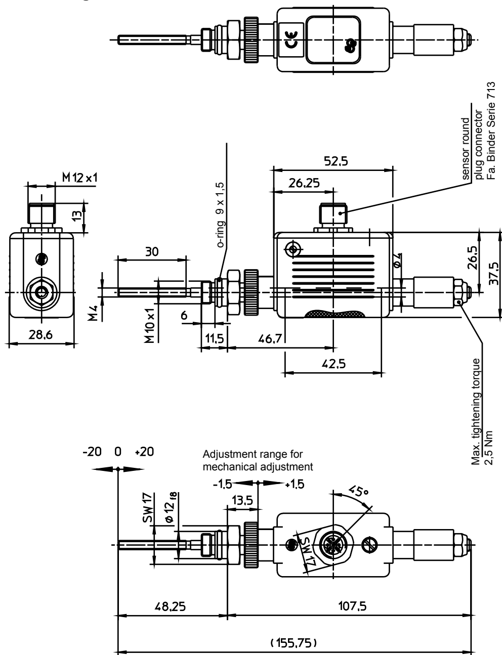
Fig. 3: Type A WE X 020 A01
